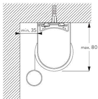
インストールレール SG 10534 & クランプ SG 3033 or SG 3044
