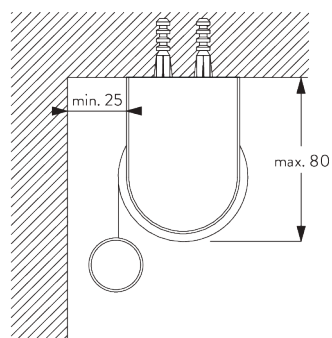
両サイドのブラケット
