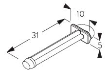
SG 10641 サイドガイドアイレット
