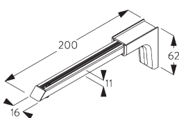
SG 11156 ユニバーサルスマートフィックス セット 200 mm
