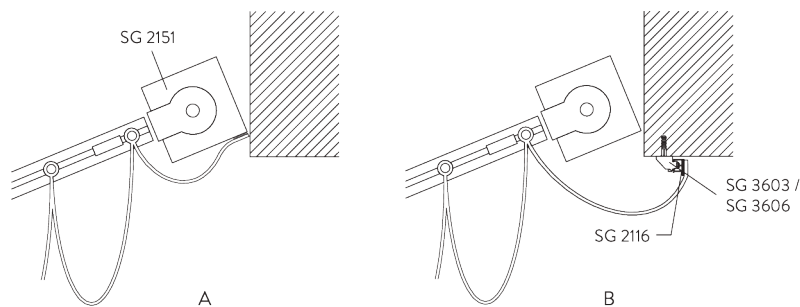
A:ファブリックをベルクロレール SG 2116 に固定 ※イラストは欧州仕様 B:ファブリックをベルクロレール SG 2116 に固定
