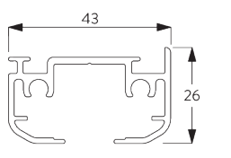
SG 2601 レール
