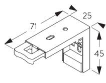
SG 8920 ブラケット
